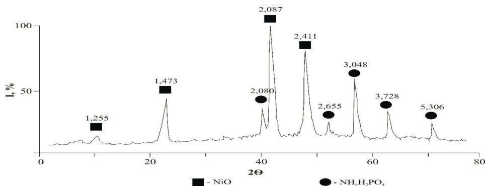
Рисунок 3 – Результат рентгенофазового анализа определения NH 4 H 2 PO 4
