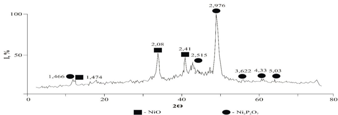
Рисунок 4 – Результат рентгенофазового анализа определения Ni 2 P 2 O 7
