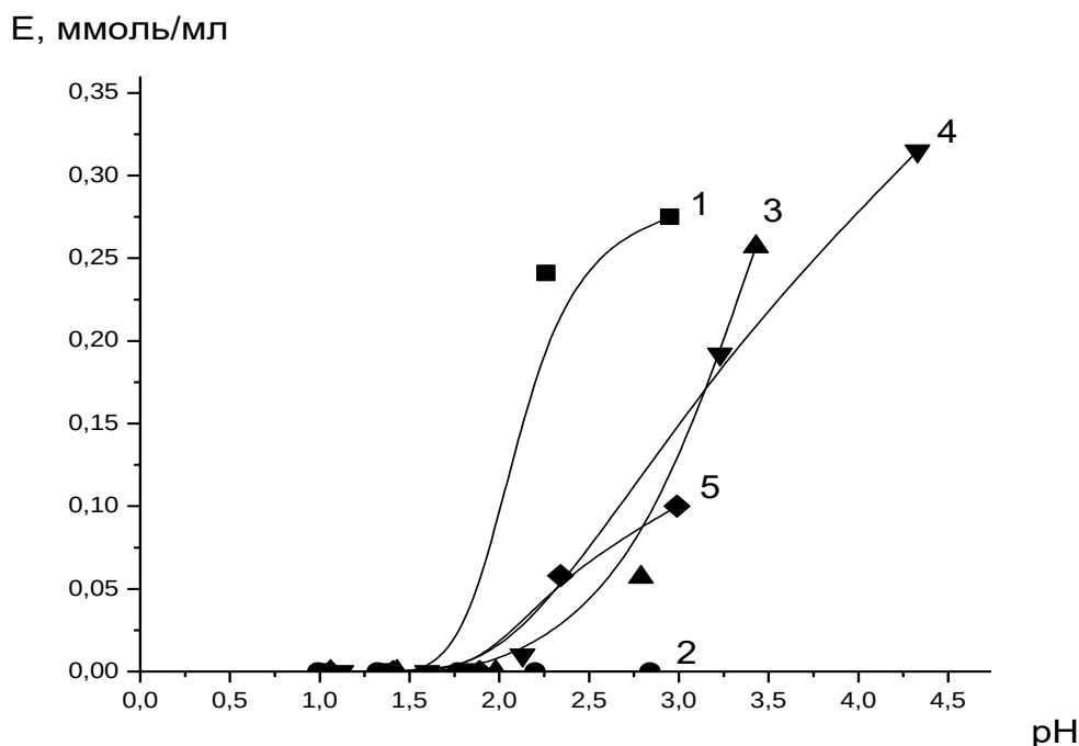
Сурет 1 – Әртүрлі иониттердегі хром бойынша pH ортасынан тәуелділік сыйымдылығы 1-топинамбур сорбенті; 2- силикагель, 3- КУ-2;4-KX-100, 5-БАУ
