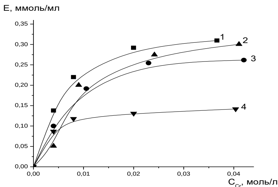
Сурет 2 - Өртүрлі иониттердегі хром(III) сорбциясының изотермасы 1-топинамбур сорбенті; 2-KX-100, 3- КУ-2; 4-БАУ
